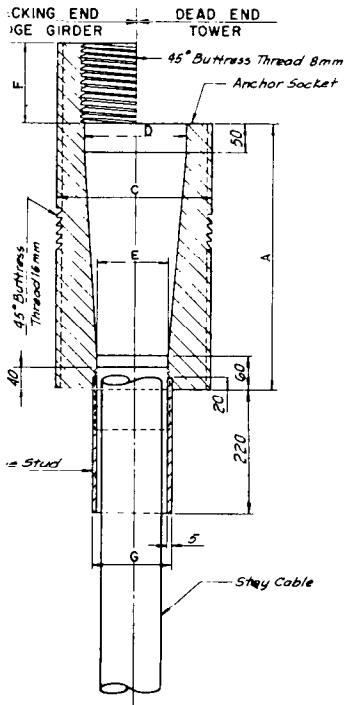
CABLE SOCKET
